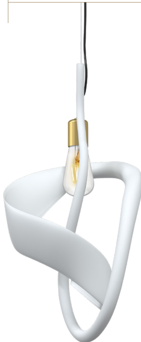
B. One Light Pendant
